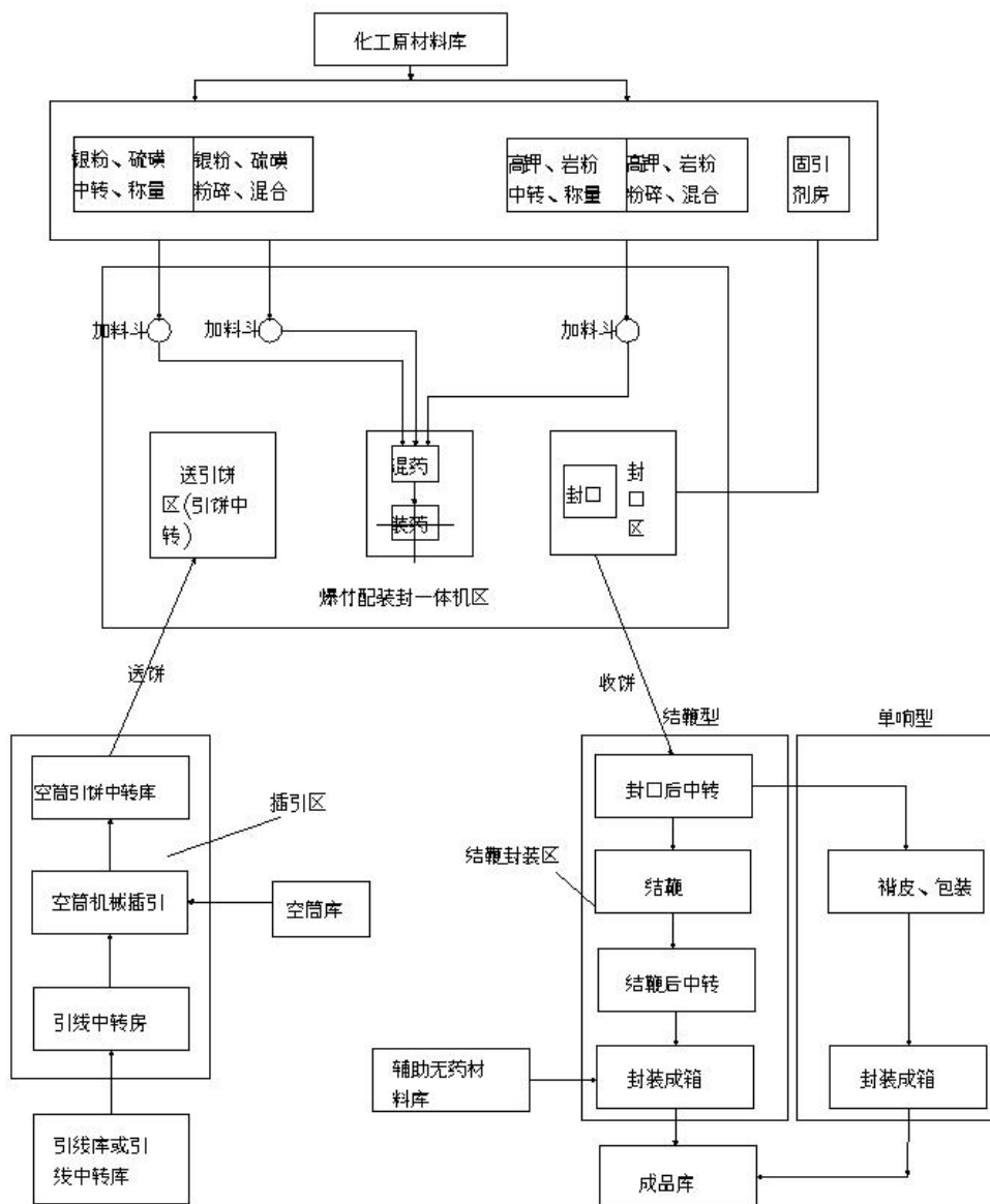
配封装一体机爆竹（白药炮）生产工艺流程图
