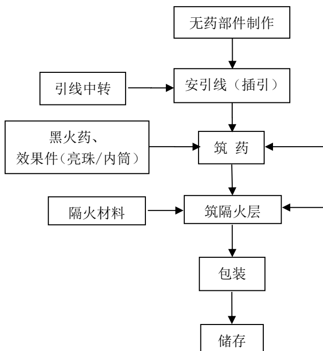
图 2.4-4 吐珠类产品生产工艺流程图
