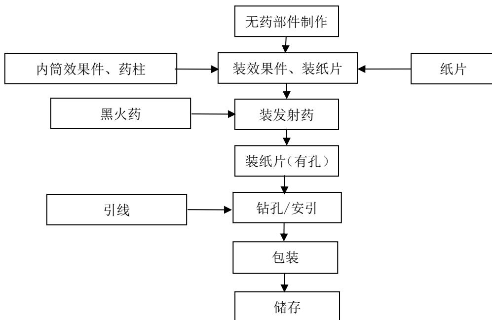
图 2.4-5 礼花类（小礼花/柱形）产品生产工艺流程图
