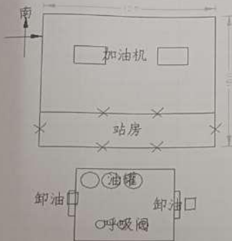
接闪器布置及保护范围图
