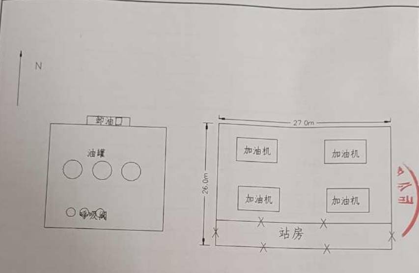
接闪器布置及保护范围图
